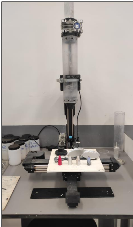
Fig. (2). 3D PotterBot 10 micro.
